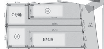
【区画図】
