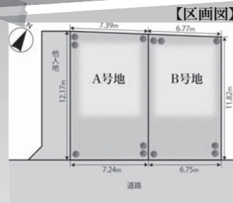
【区画図】
