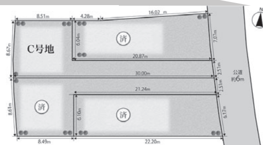
【区画図】
